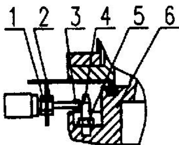
Схема №15 Регулировка микровыключателя загрузочного люка.
