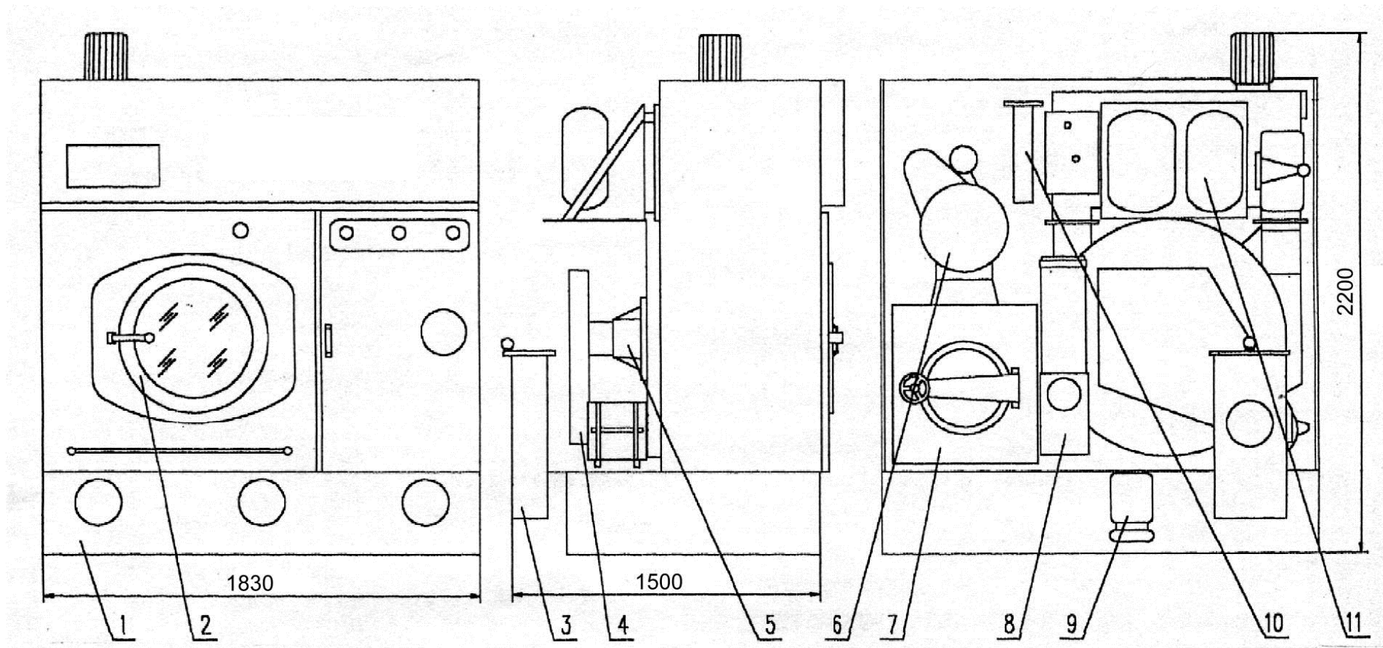
Рис. 1 Общий вид машины сухой чистки ЛВХ-16
