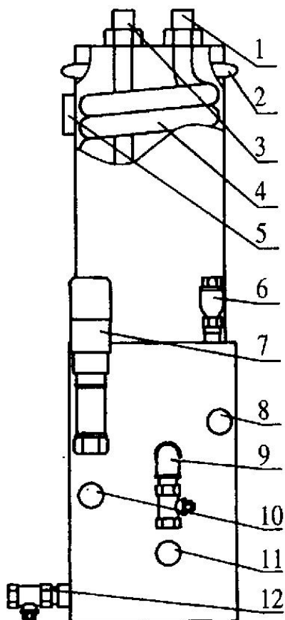
Схема №9 Охладитель дистиллята и отделитель воды.
