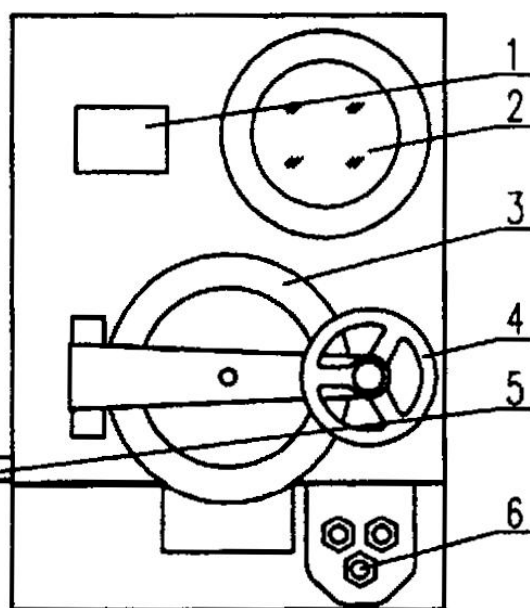
Схема №13 Дверца дистиллятора.
