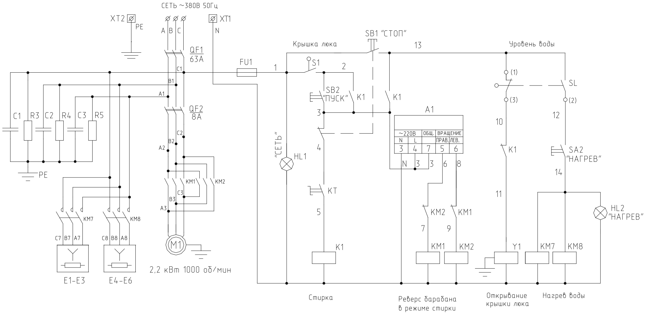
Рис.3а. Схема электрическая принципиальная машины стиральной Л60-121
