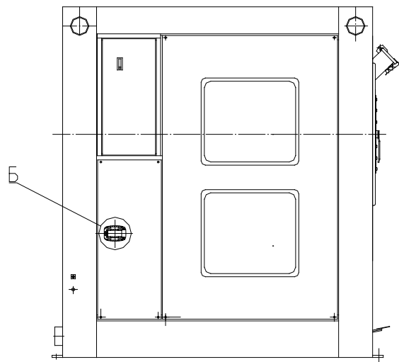
Рис.7 Схема смазки. 1.Подшипники промежуточной опоры. 2.Оси загрузочного люка. 3.Ригель замка загрузочного люка. 4.Ось замка загрузочного люка.
